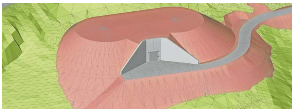
3D-Ansicht des künftigen Hochbehälters (Adler+Partner ZT GmbH) – sichtbar bleiben nach Fertigstellung nur die grauen Bereiche.
